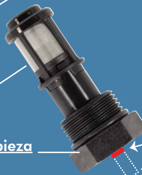
Posición del indicador para el filtro vacío
